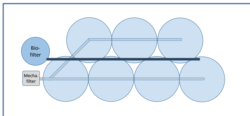
A halnevelő modellrendszer elvi elhelyezése a 22,5 x 10 m méretű, 2,9 m oldalfal-magasságú egyhajós dupla felfűjt borítású fóliasátorban
