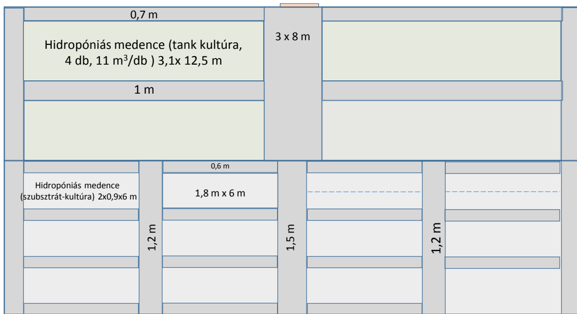
A hidropóniás medencék elvi elhelyezése a 2x8x30 m méretű, 2,3 m oldalfal-magasságú kéthajós dupla felfűjt borítású fóliasátorban
