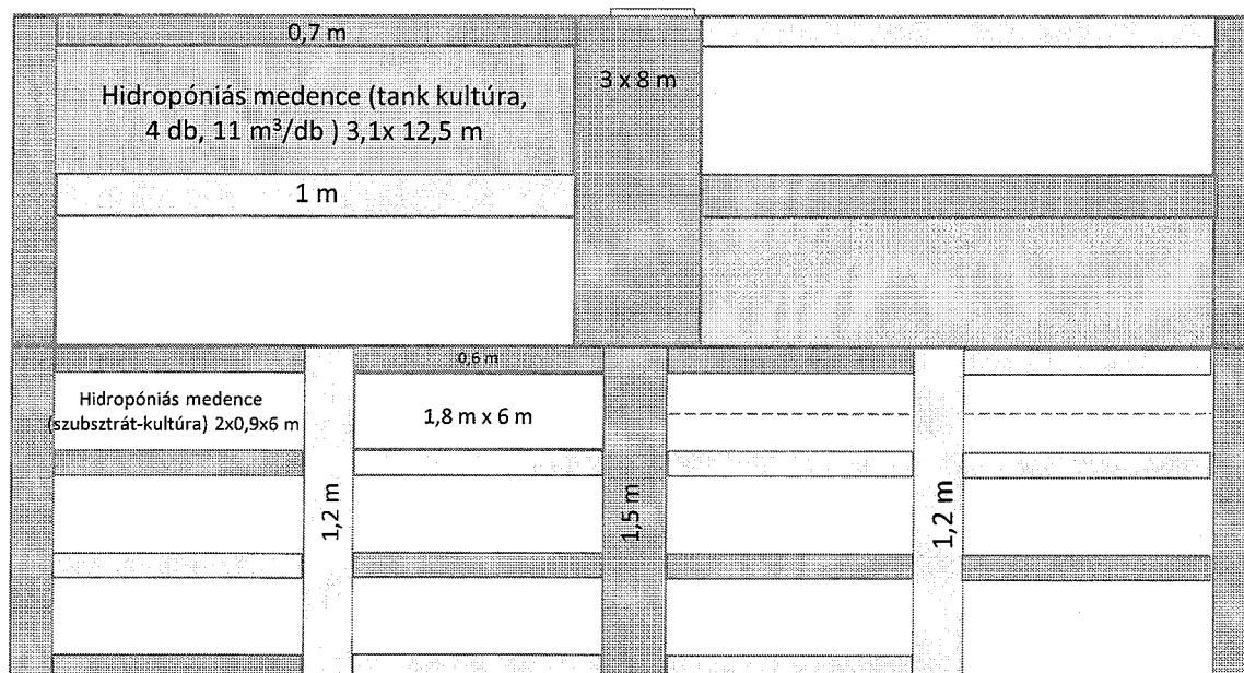
A hidropóniás medencék elvi elhelyezése a 2x8x30 m méretű, 2,3 m oldalfal-magasságú kéthajós dupla felfújott borítású fóliasátorban
