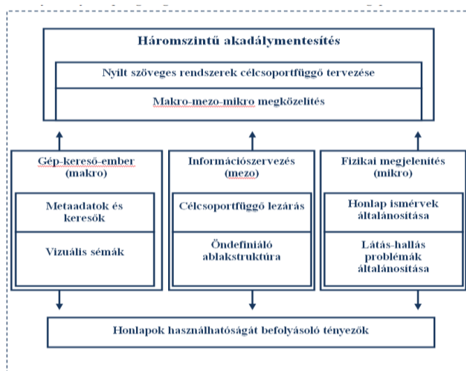
15. ábra Honlapok háromszintű akadálymentesítése
